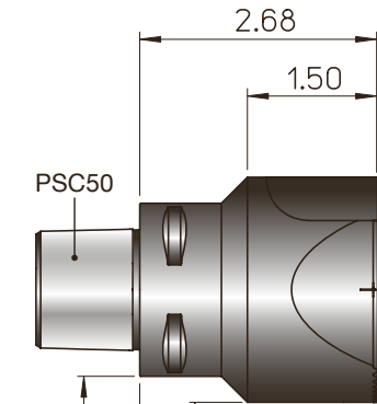
PSC50 - TS50 \varnothing 2.68 ~ 3.54
