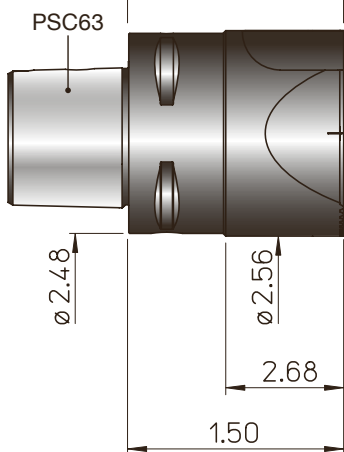
PSC63 - TS50 \varnothing 2.68 ~ 3.54
